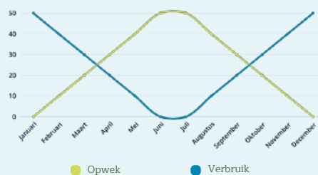
Energieverbruik en -opwek over één jaar
