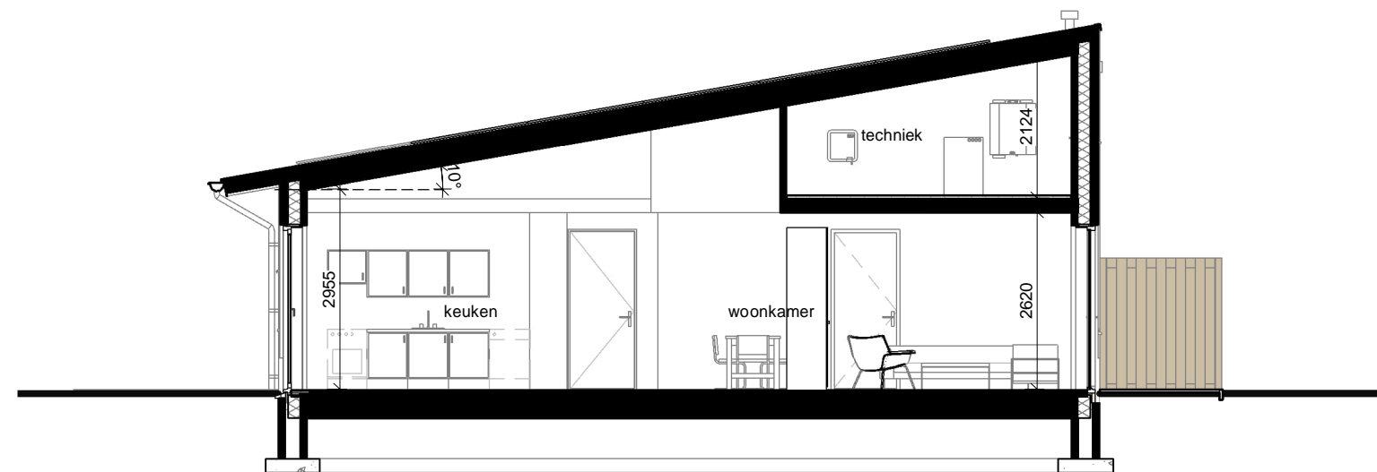
dwarsdoorsnede
