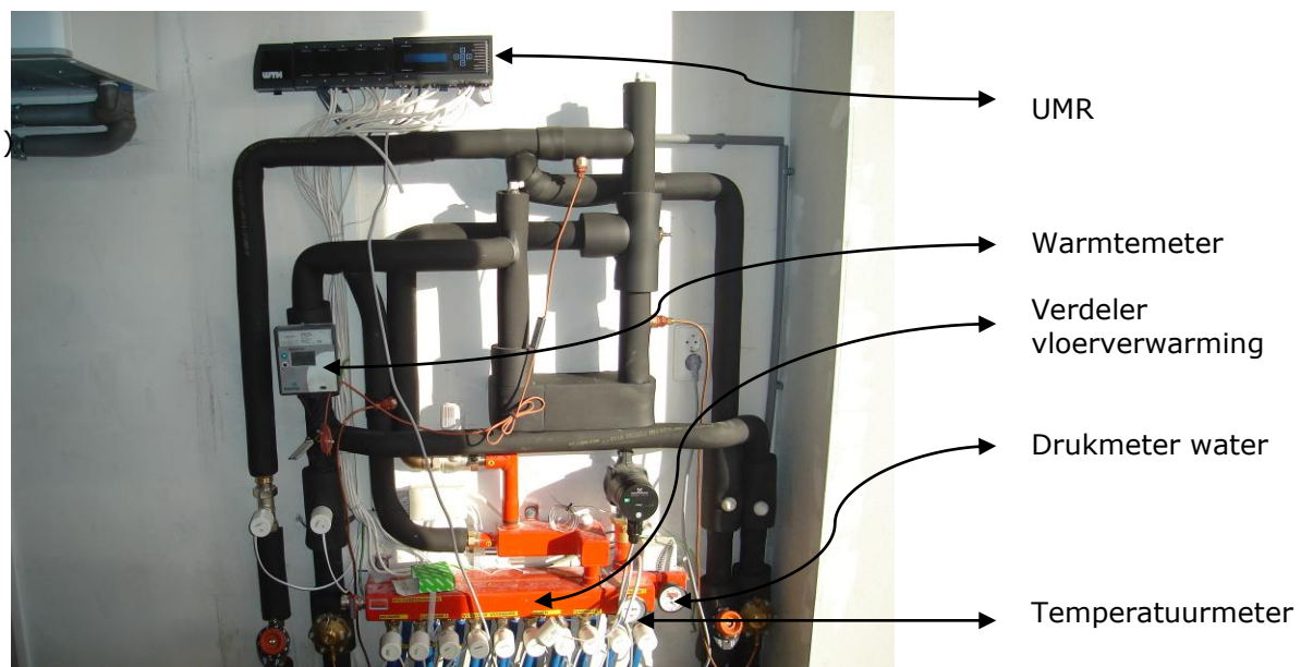
Foto verdeler vloerverwarming
